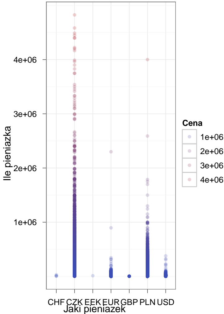
Koszt vs Waluta?
