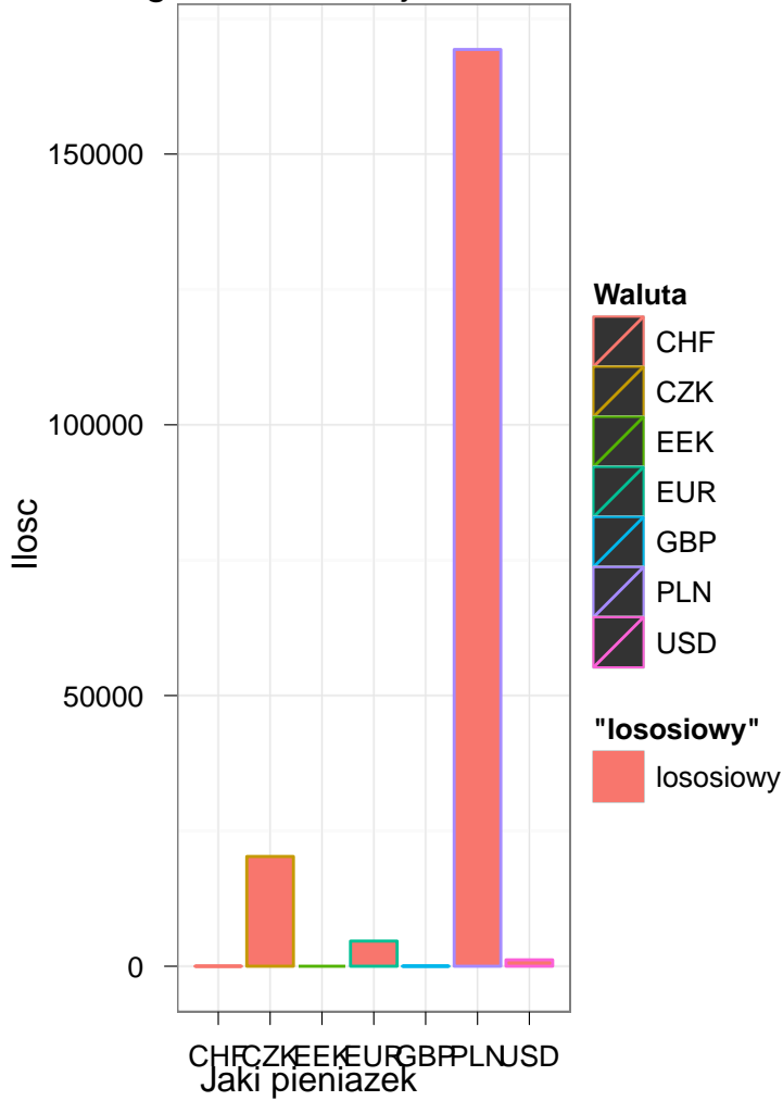
Histogram zmiennej 'Waluta'
